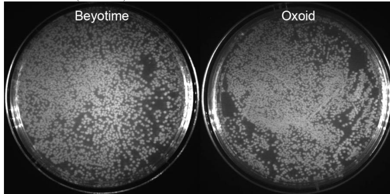
图1. 碧云天的BeyoPure™ LB Broth with Agar (premixed powder)配制的LB琼脂培养基与用国外Oxoid的胰蛋白胨和酵母膏配制的LB琼脂培养基, 培养的大肠杆菌DH5 \alpha 菌落形态图。培养条件和培养时间完全相同。
